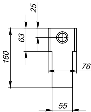
Поз.5 (Пластина)
