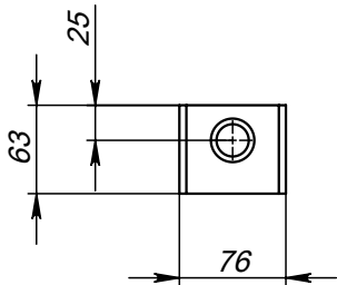
Поз.4 (Пластина)
